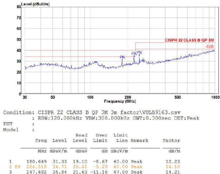
图 5-5 RE 测试水平方向
