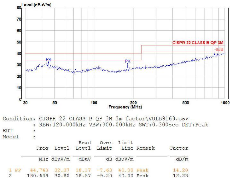
图 5-6 RE 测试垂直方向
